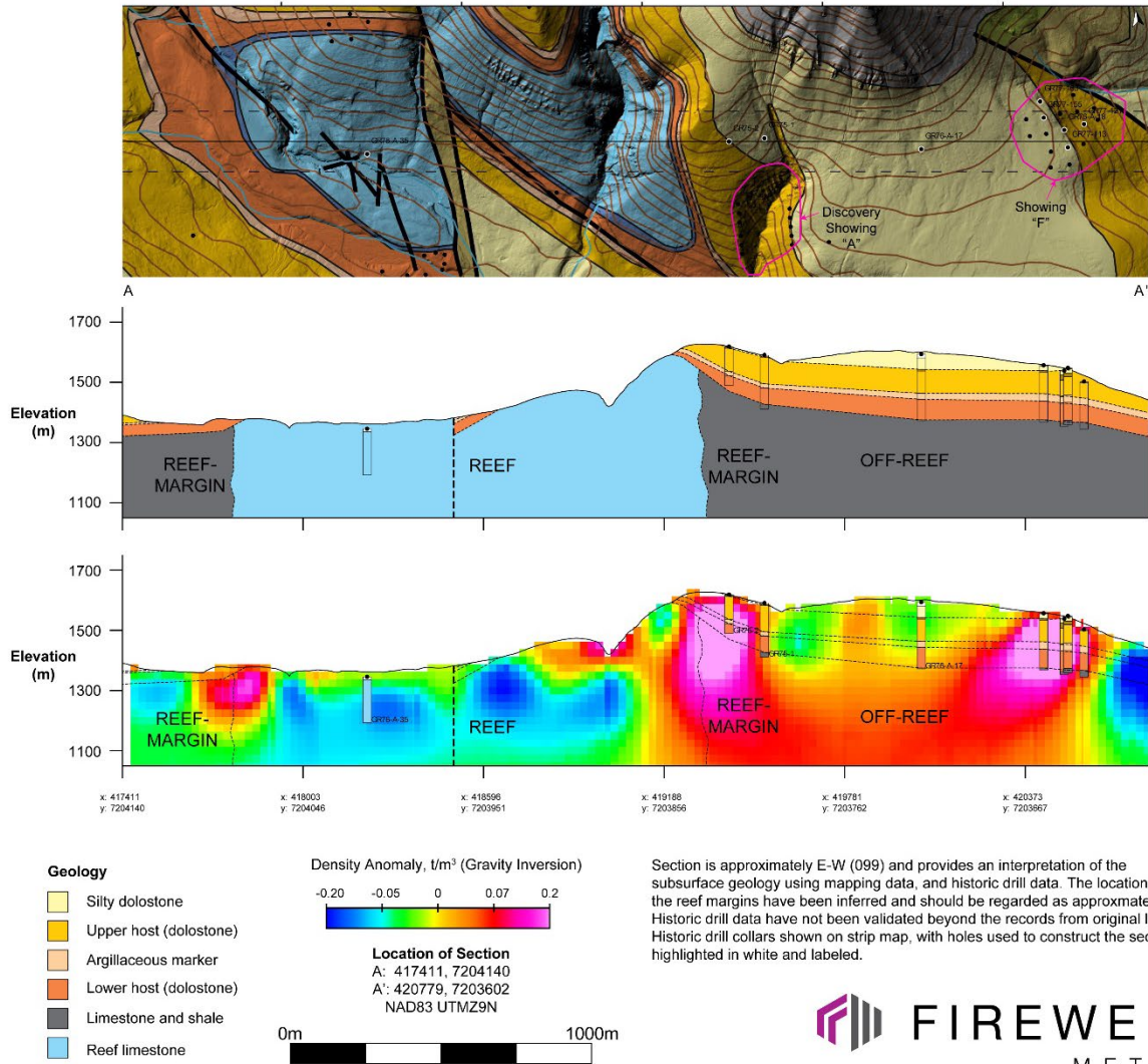
Section A-A'
